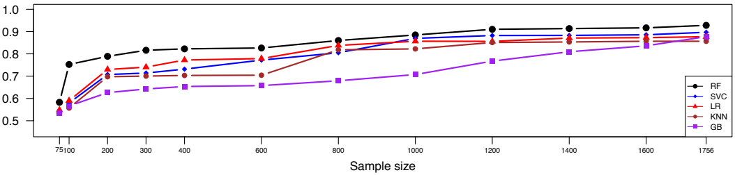
(b) Standard AUC
